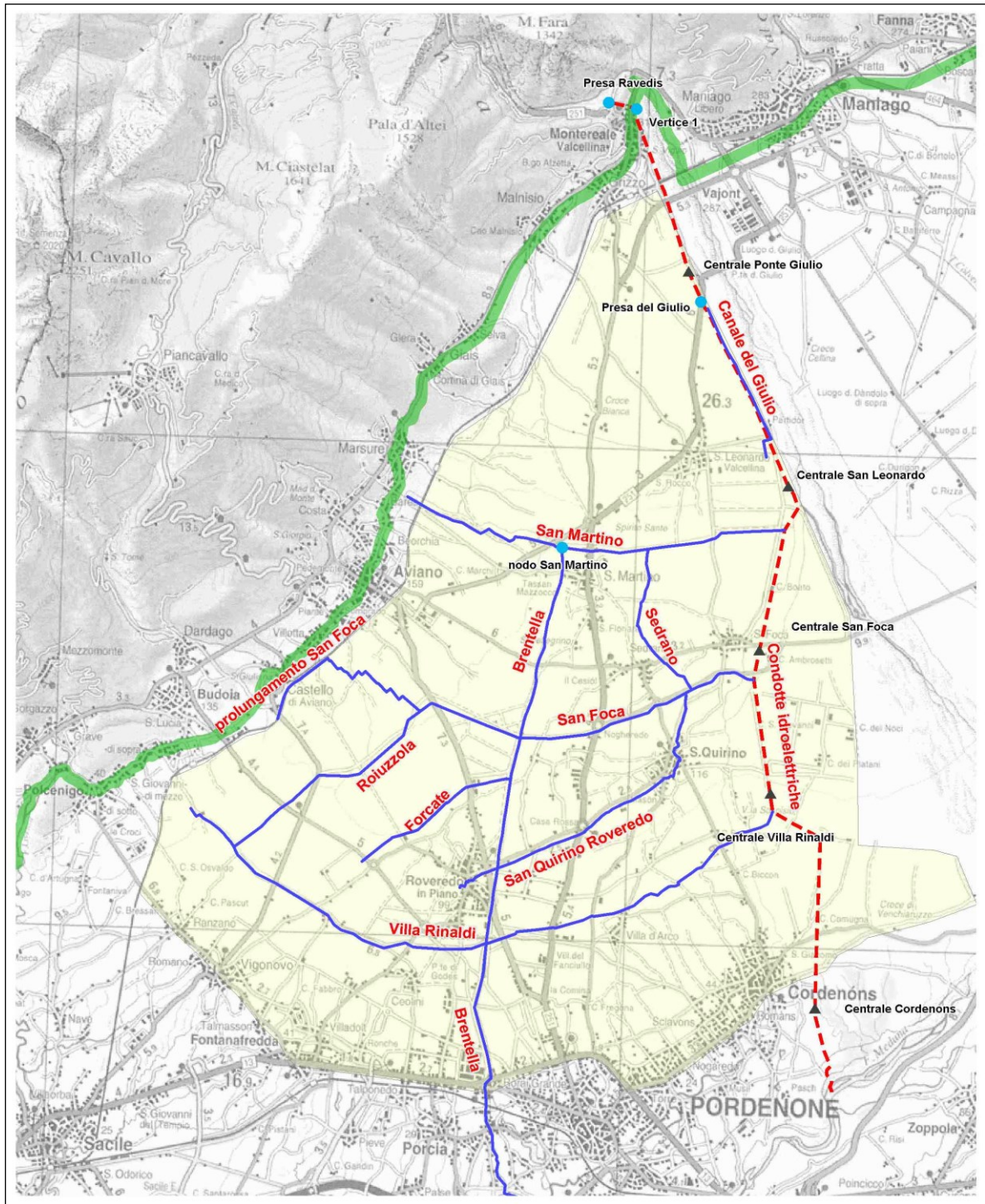
Figura 7 - Schema dei canali principali della zona Cellina
